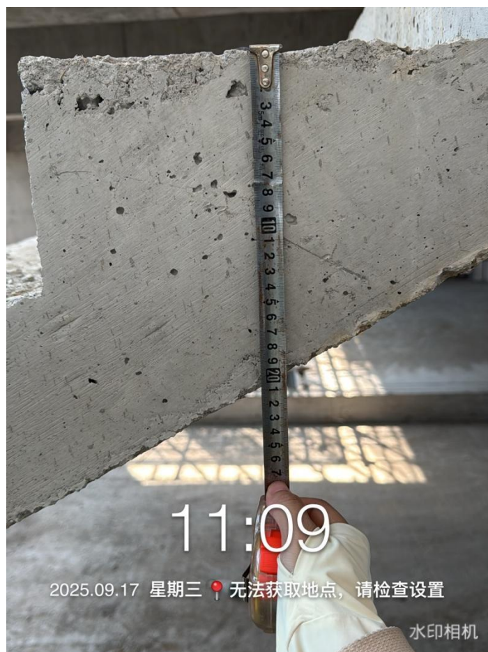
楼梯厚度测量
