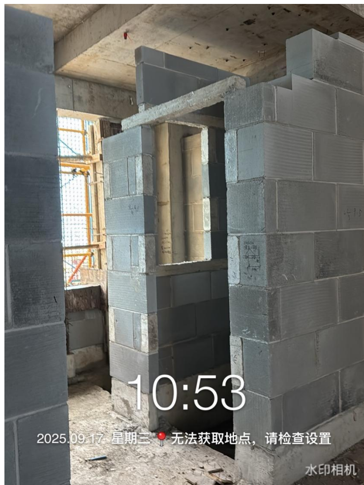
卫生间过梁
