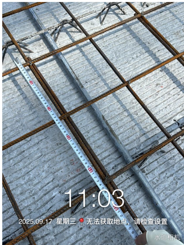
钢筋搭接长度测量
