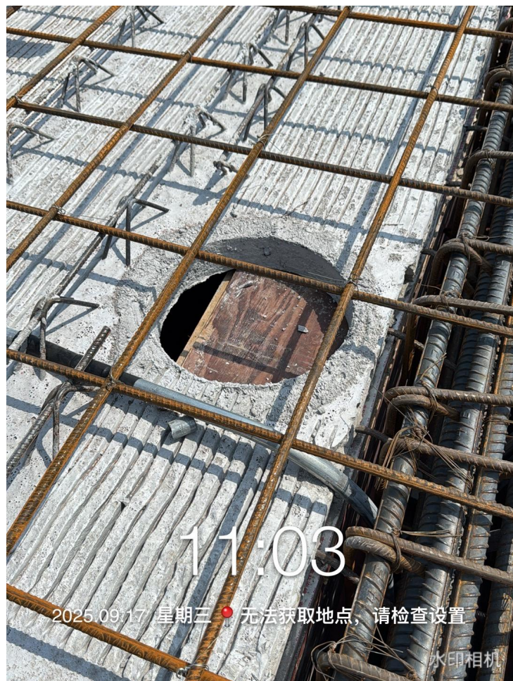
洞口钢筋照片
