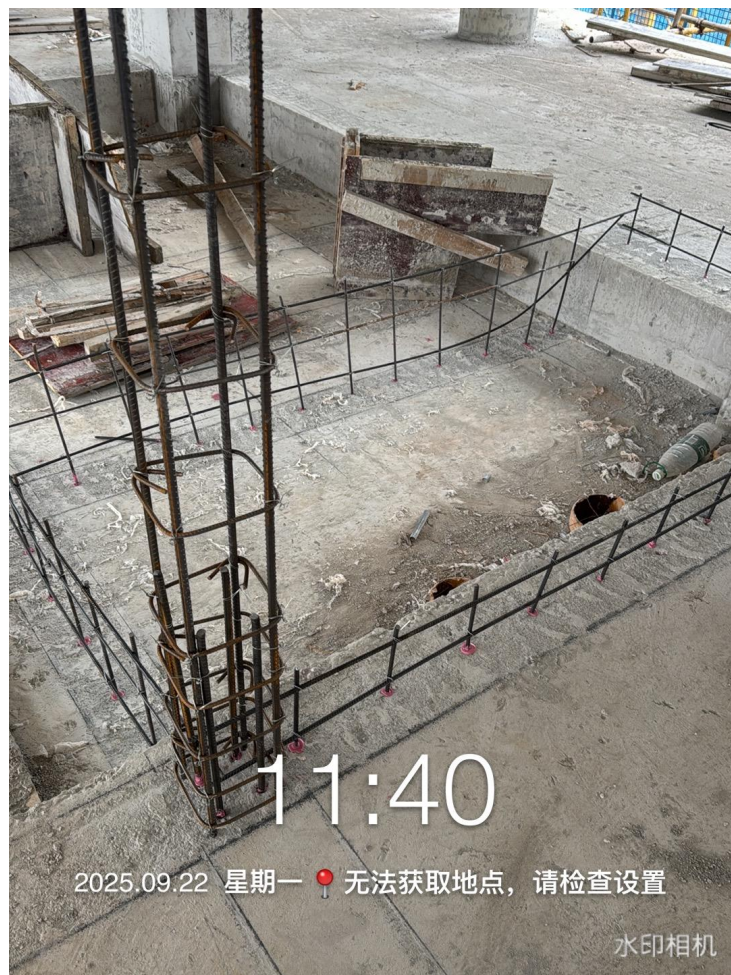
宿舍 3 层以上水电井反坎处布置钢筋
