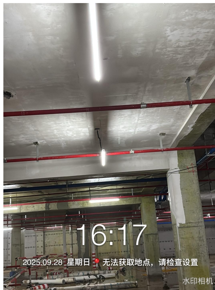
地下室乳胶漆天棚, 刷低固刮腻子
