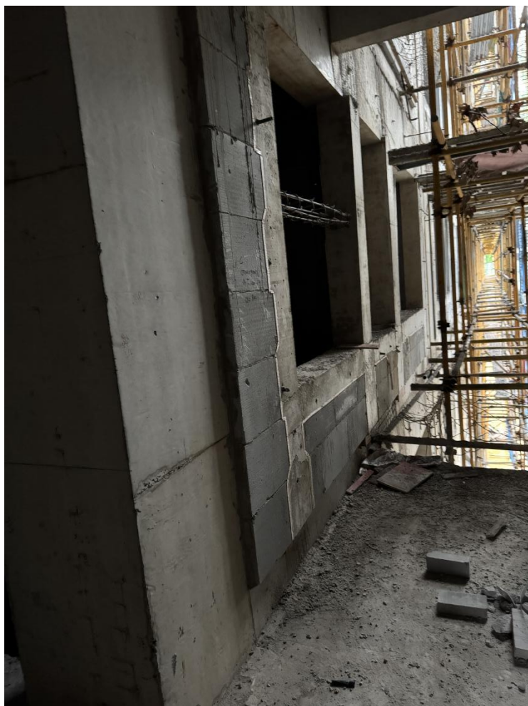
2 号楼 2 层自保温外墙（保温墙厚 250mm，反坎宽度 200mm）
