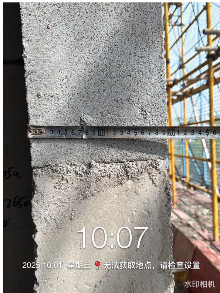
3 号楼外墙厚度测量
