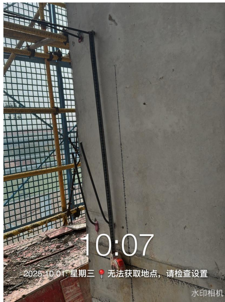
3 号楼外墙砌体植筋间距测量
