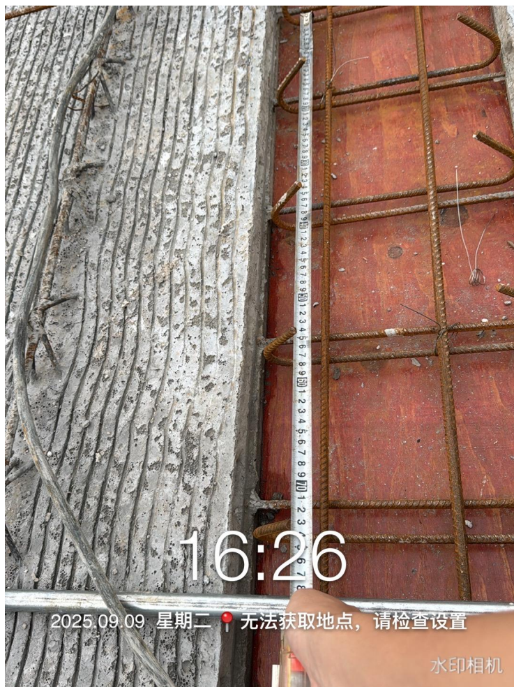
叠合板钢筋测量
