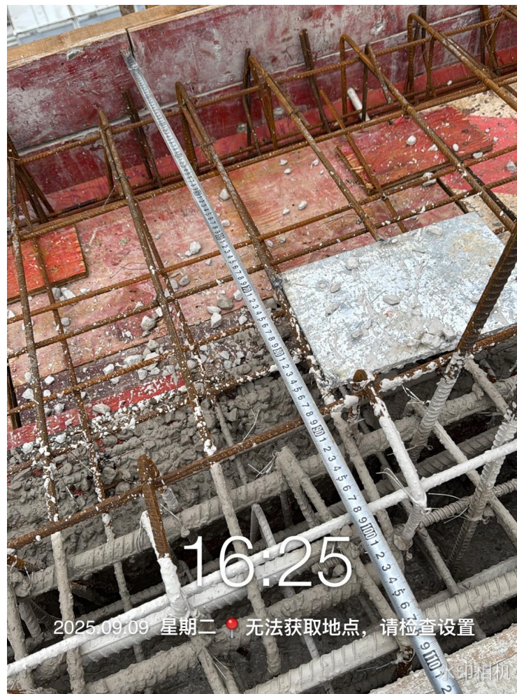
1 号楼 6 层挑板宽度测量
