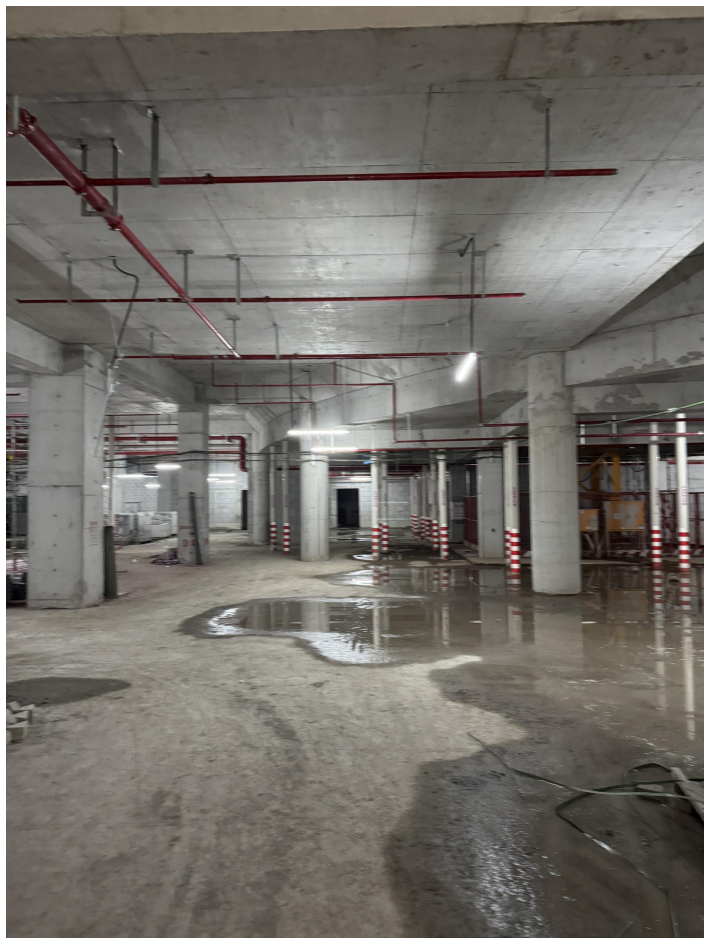
地下室消防施工
