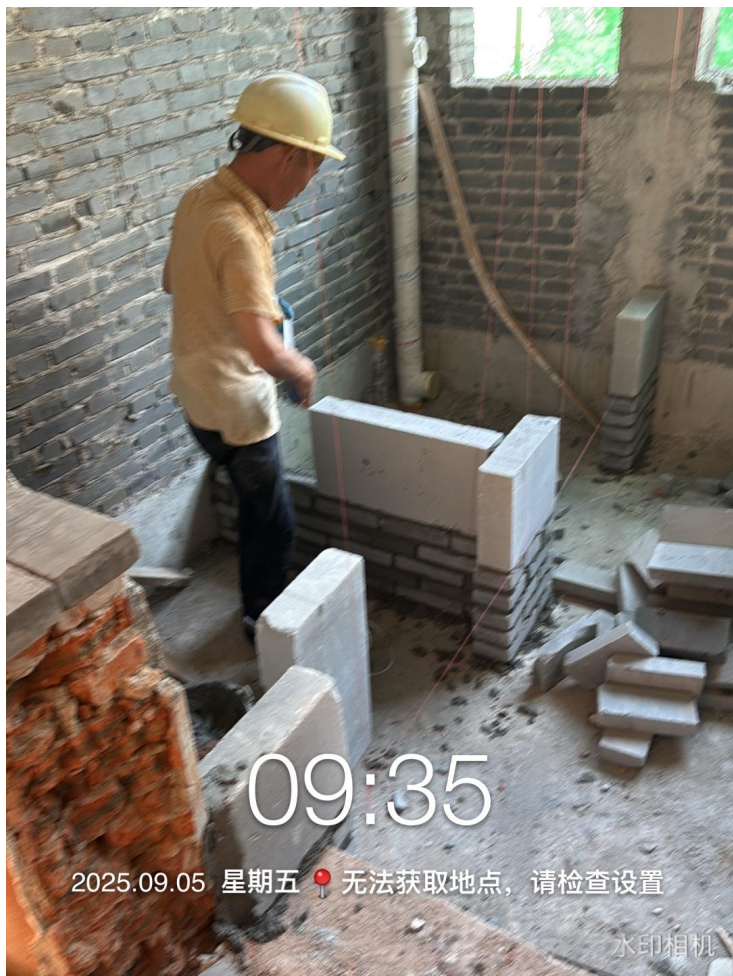
卫生间内隔墙测量
