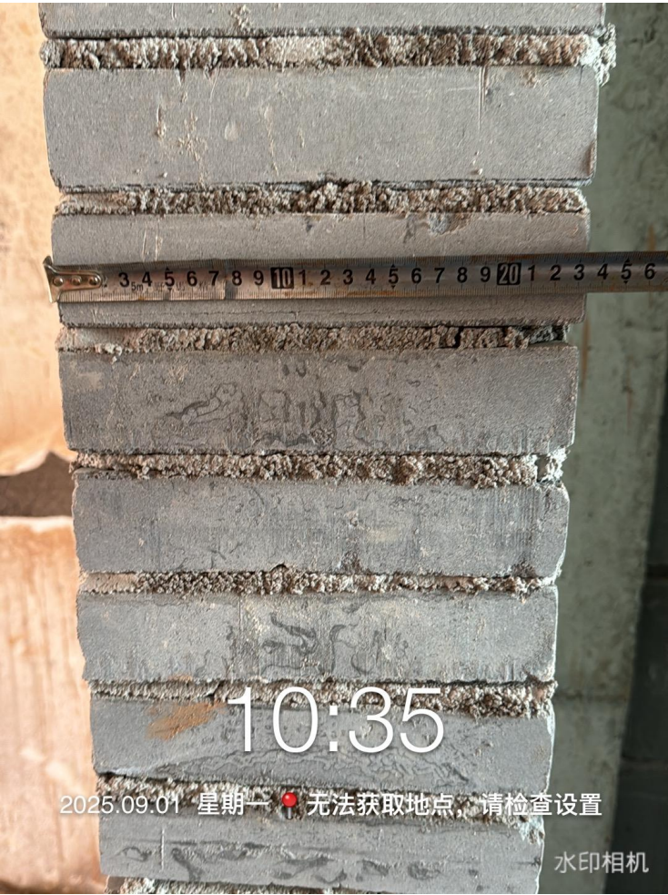
卫生间门侧砌筑测量
