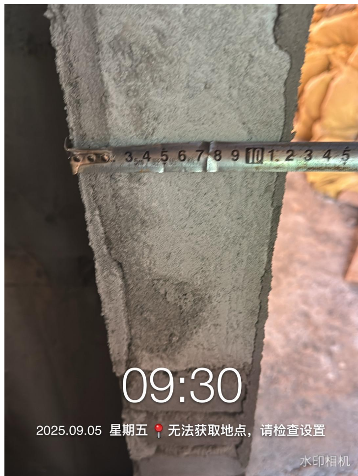
卫生间内隔墙抹灰厚度测量
