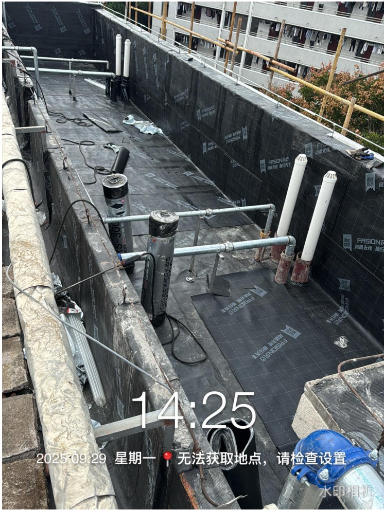
新建屋面第二道防水卷材施工
