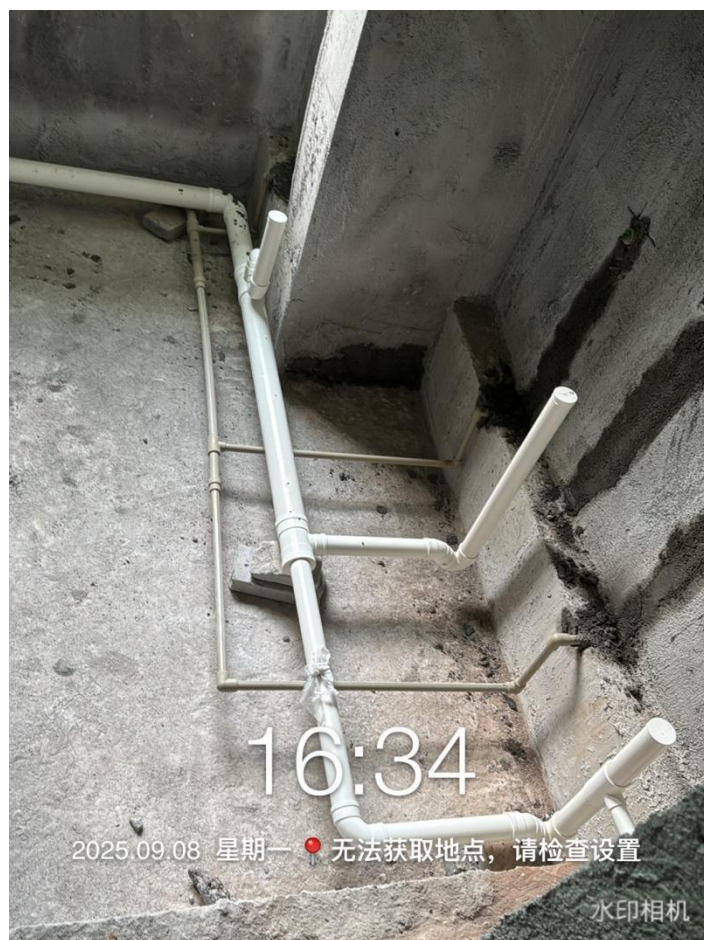
水管及管件材料进场（材料品牌为联塑）
